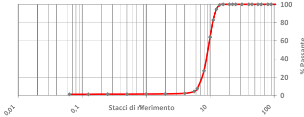
Curva Granulometrica Tipica - Carta Semilogaritmica
